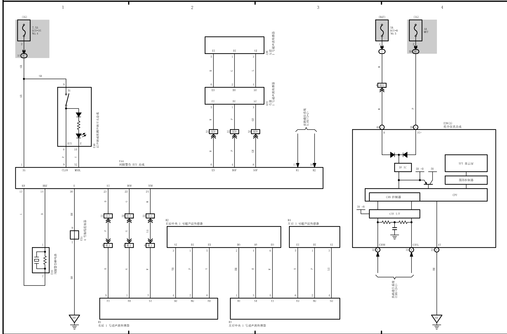
丰田驻车辅助传感器系统
